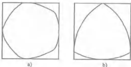
图 4.7 给定直径的曲线的最大长度
