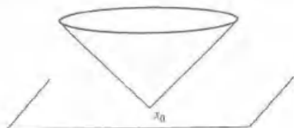
图 6.3 起始于 (x, t) 的前光锥
