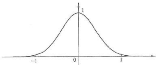
图 5.1 高斯函数 e^{-\pi x^2}
