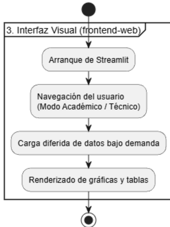
Figura C.8: Diagrama de actividad del módulo de Interfaz Visual
