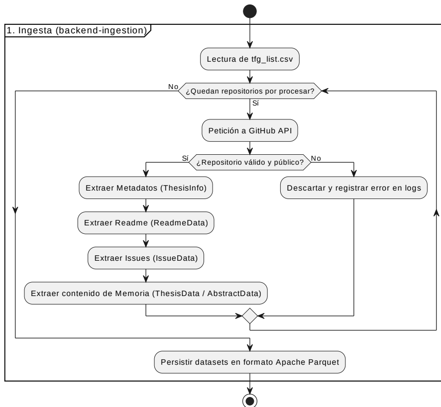
Figura C.4: Diagrama de actividad de la fase de Ingesta
