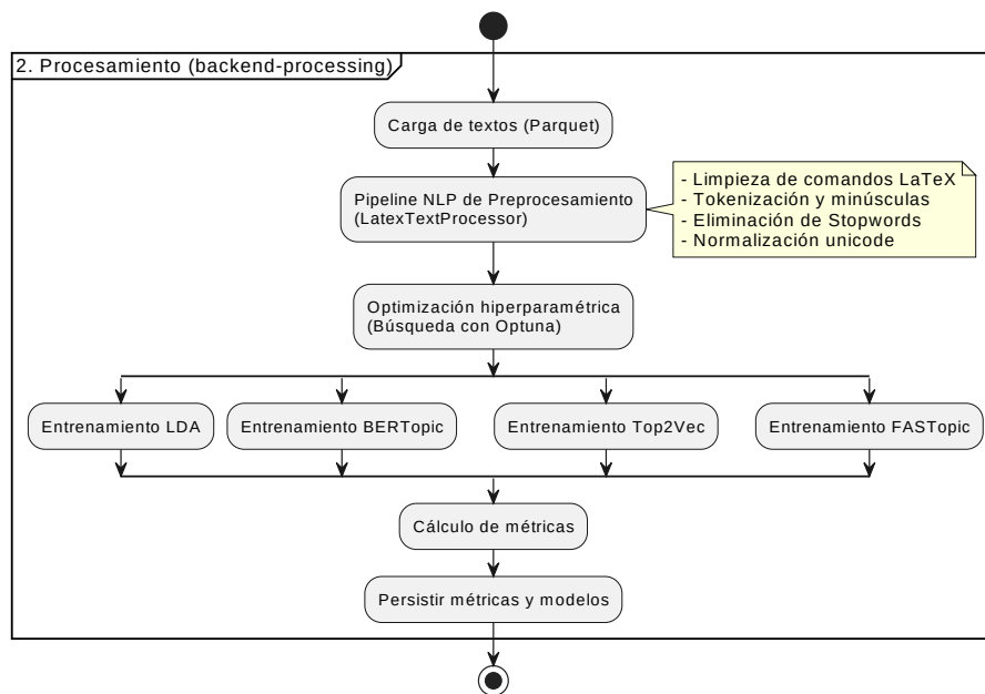
Figura C.6: Diagrama de actividad de la fase de Procesamiento
