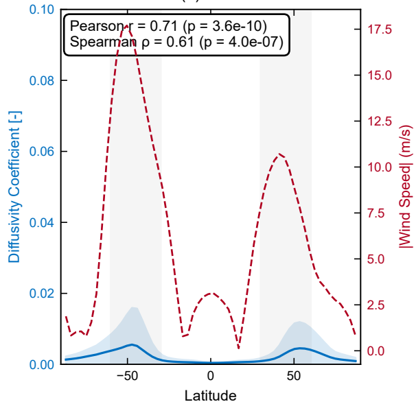
(b) LGM
