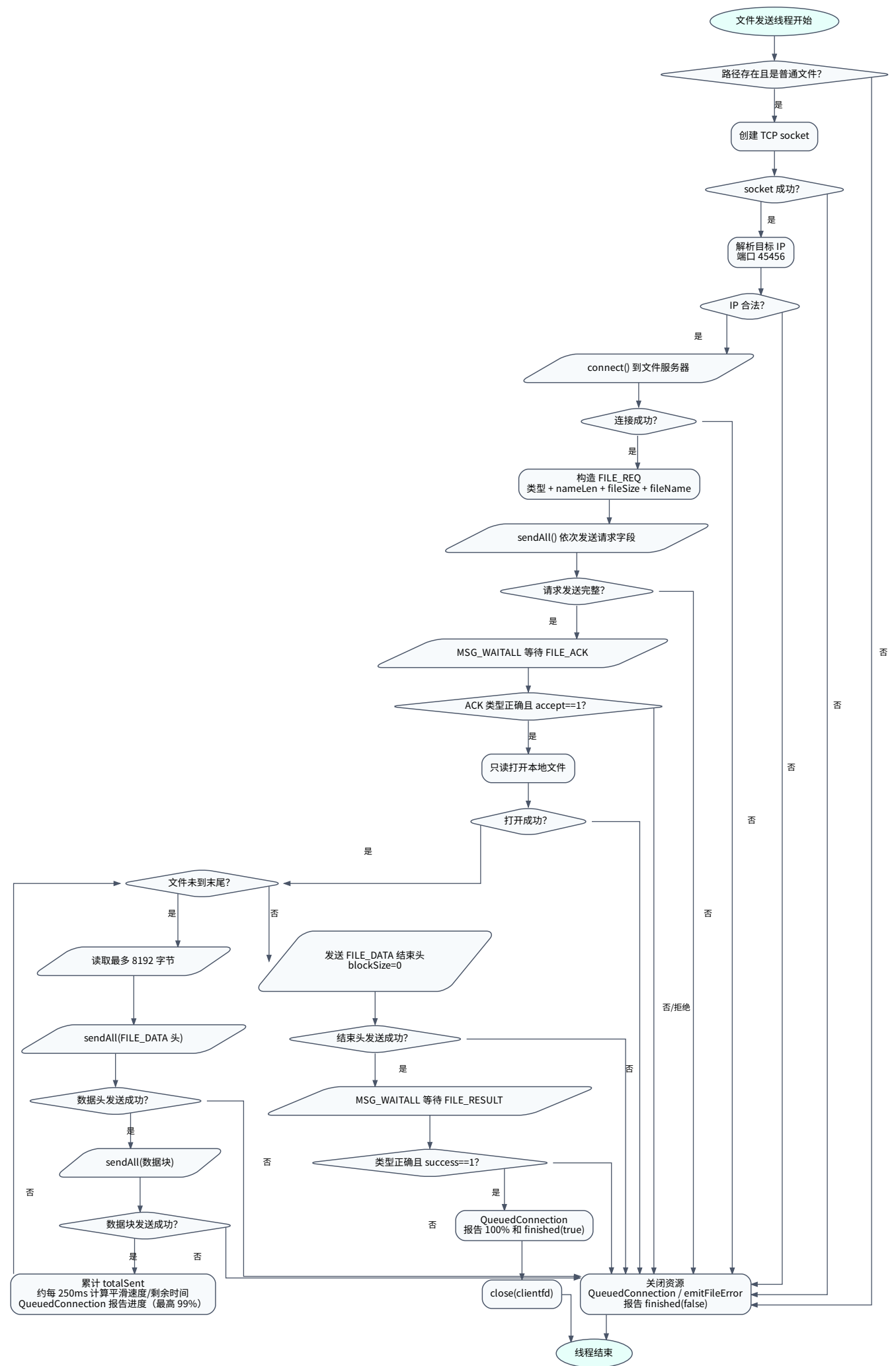
13 TranslateFile - 文件发送线程流程图
