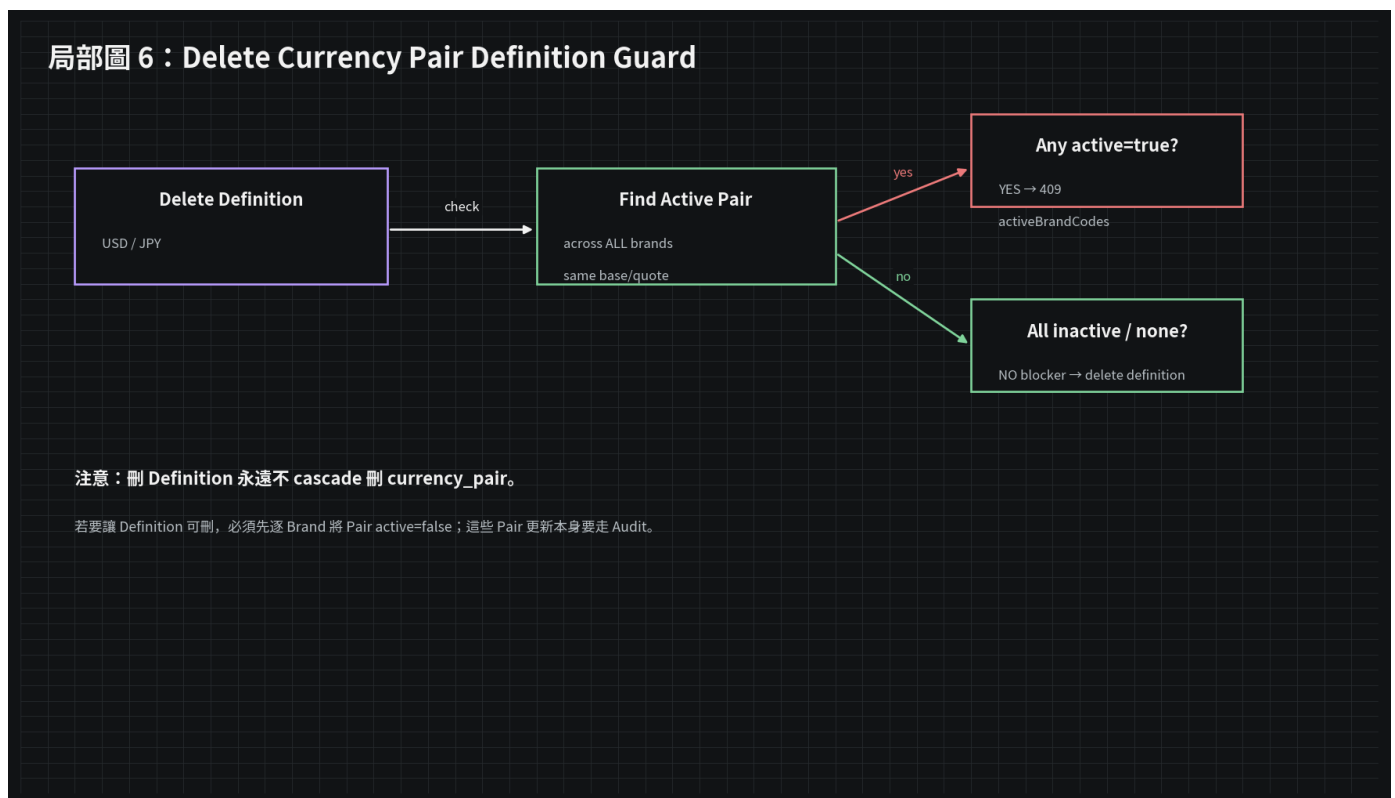
圖 3 - Definition DELETE 前必須保證所有 Brand 的同方向 Pair 都 inactive
