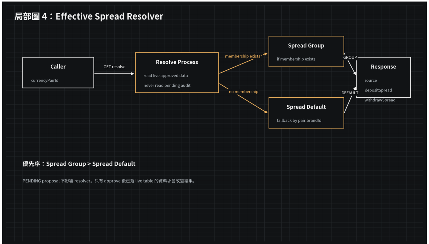
圖 7 - Runtime Spread 選擇：Group 優先，Default fallback
