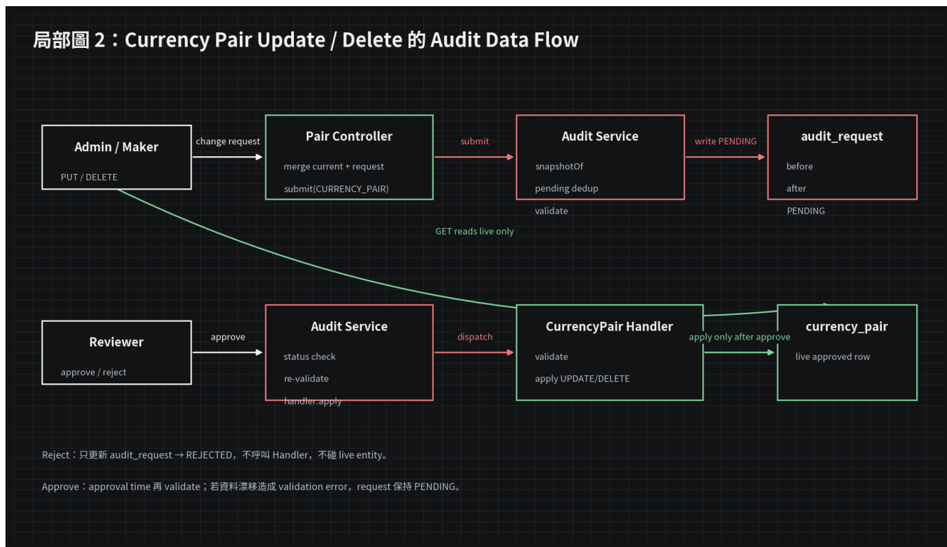
圖 4 - Currency Pair 更新／刪除不直接寫 live table
