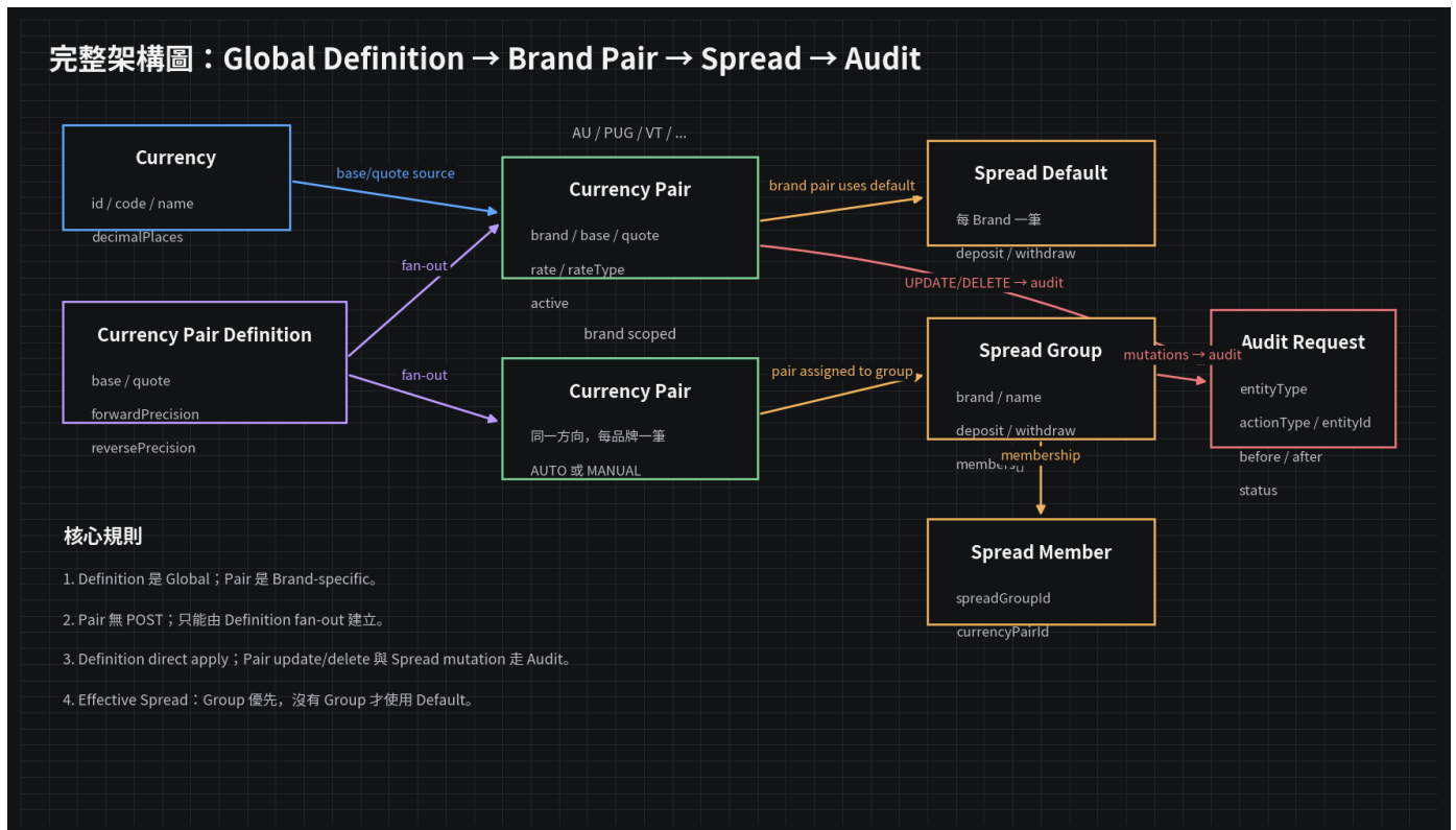
圖 1 - 完整架構：資料主檔、Global Definition、Brand Pair、Spread 與 Audit
