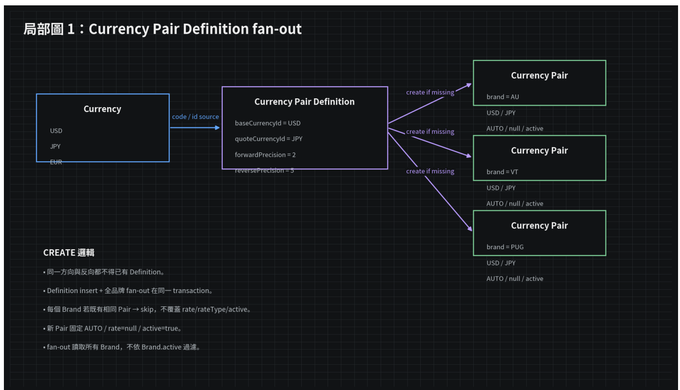
圖 2 - Global Definition 建立後 fan-out 到每一個 Brand
