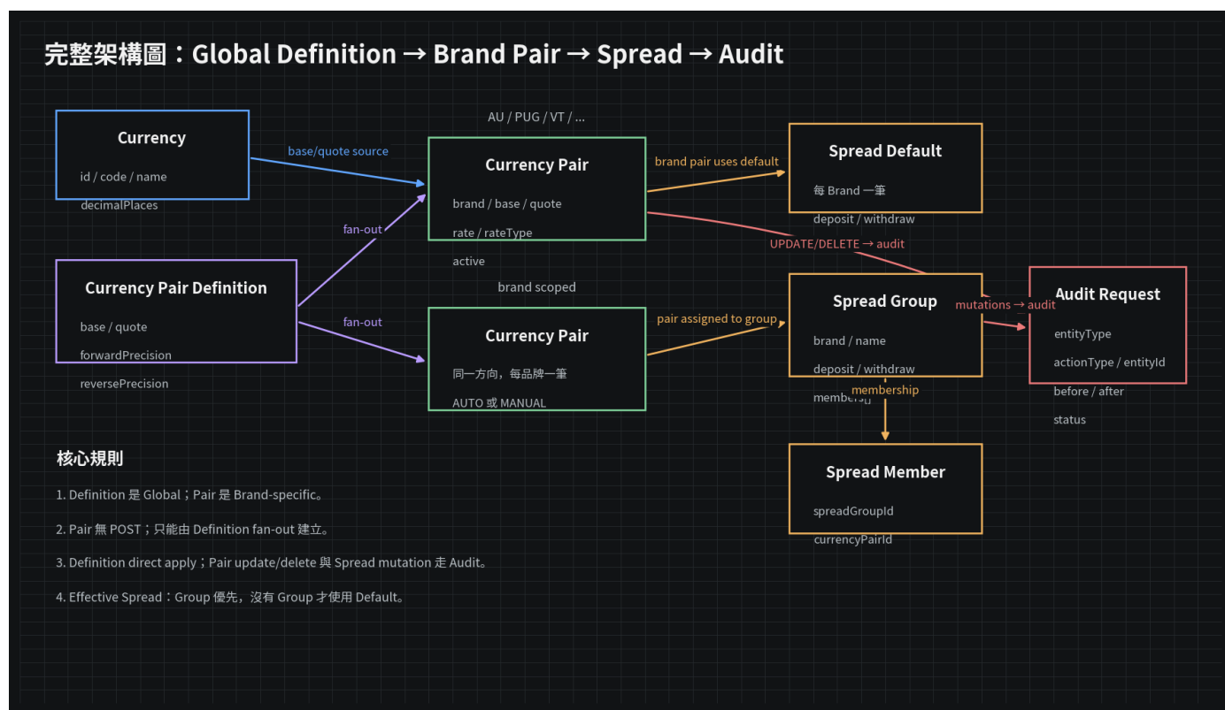
圖 0 - 完整架構總覽
