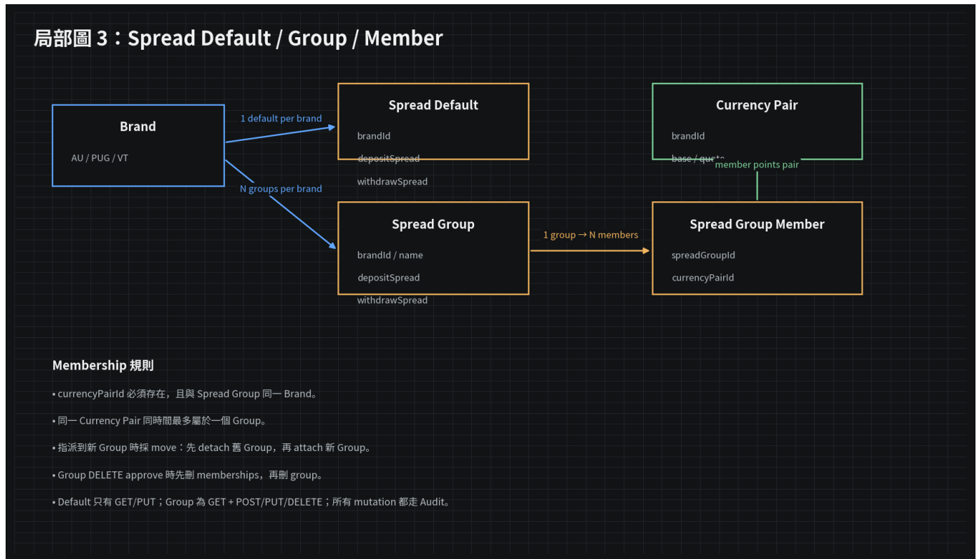
圖 6 - Spread 的三個 live data structures
