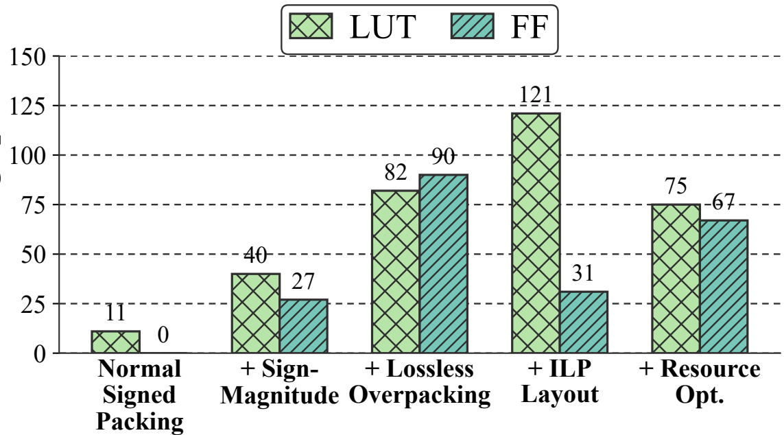
Resource Usage per DSP
