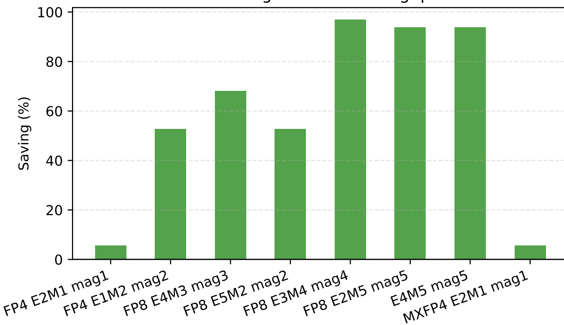
D. LUT Saving vs Same-Throughput LUT
