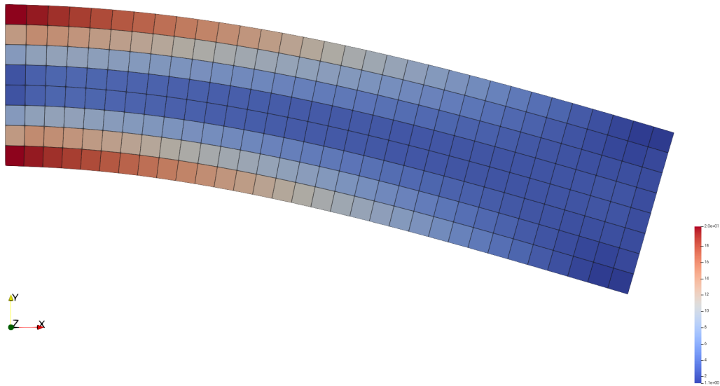
图 4 悬臂梁 32×8 网格的变形图与平面应力 von Mises 云图（位移放大 3 倍）。
