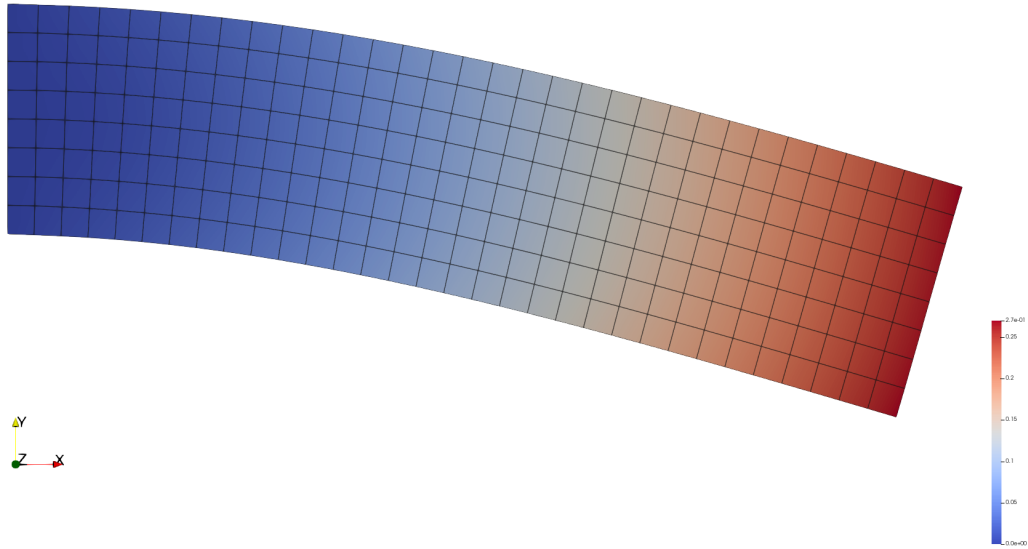
图 3 悬臂梁 32×8 网格的变形图与位移模量云图（位移放大 3 倍）。
