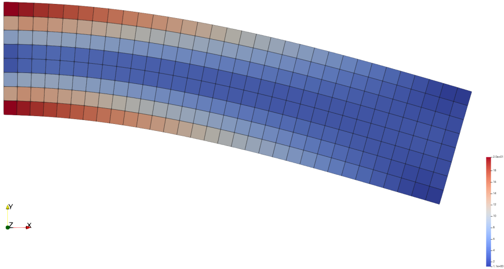
图 3 悬臂梁 32×8 网格的变形图与平面应力 von Mises 云图（位移放大 3 倍）。
