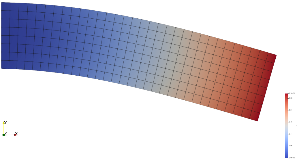
图 2 悬臂梁 32 \times 8 网格的变形图与位移模量云图（位移放大 3 倍）。
