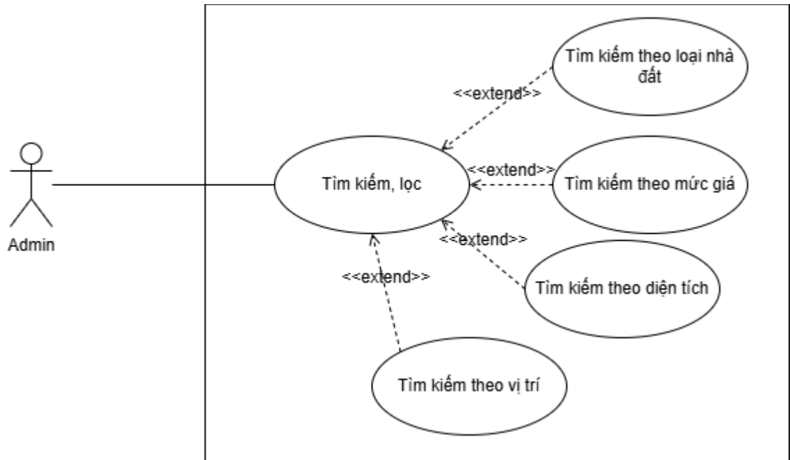
Hình 2.16 Sơ đồ Usecase Tìm kiếm, lọc
