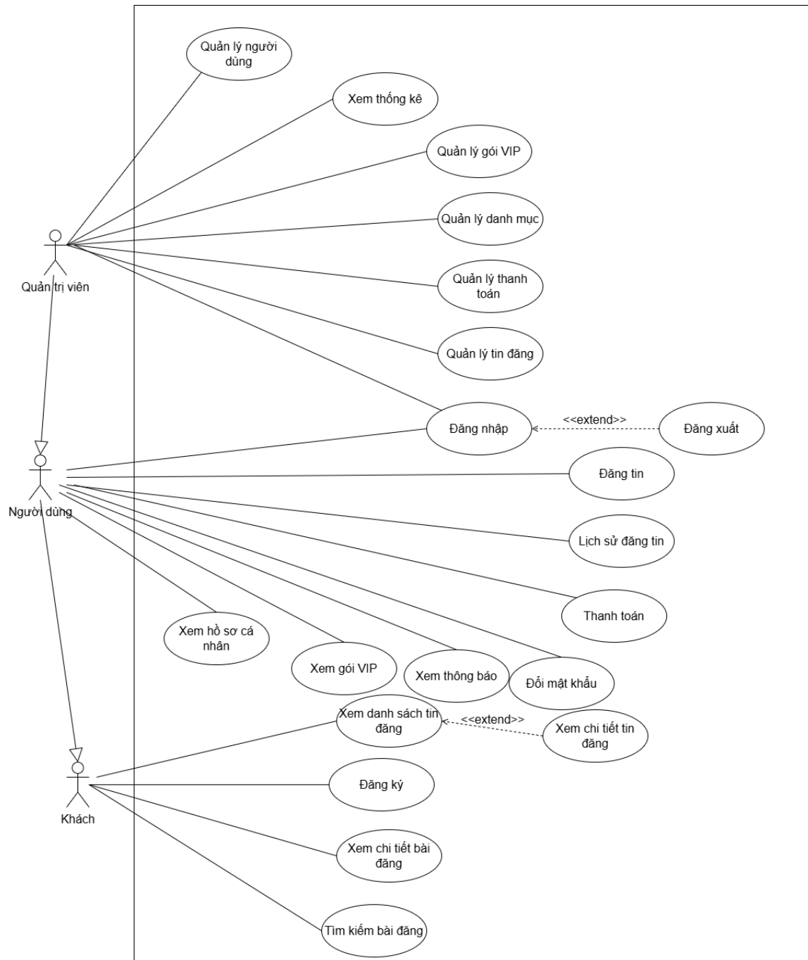
Hình 2.1 Usecase Tổng quát
