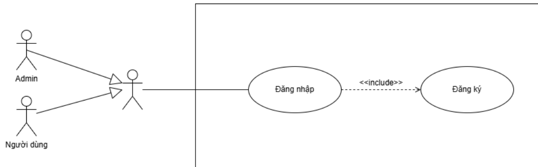
Hình 2.2 Sơ đồ Usecase Đăng nhập
