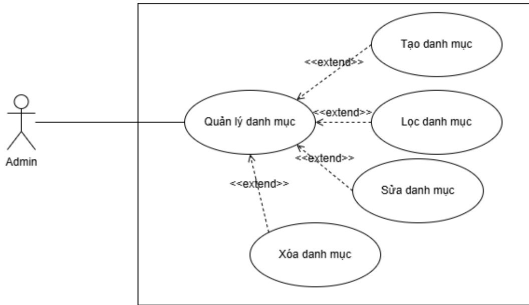
Hình 2.15 Sơ đồ Usecase Quản lý danh mục
