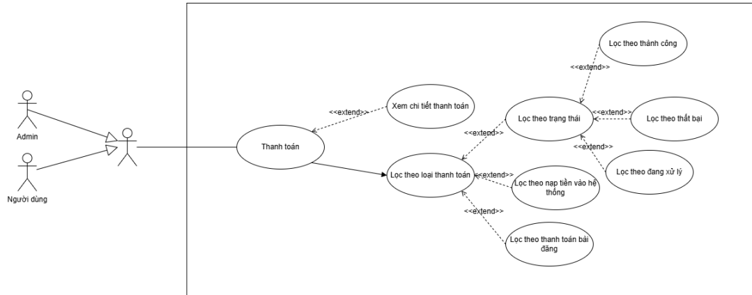
Hình 2.8 Sơ đồ Usecase Thanh toán
