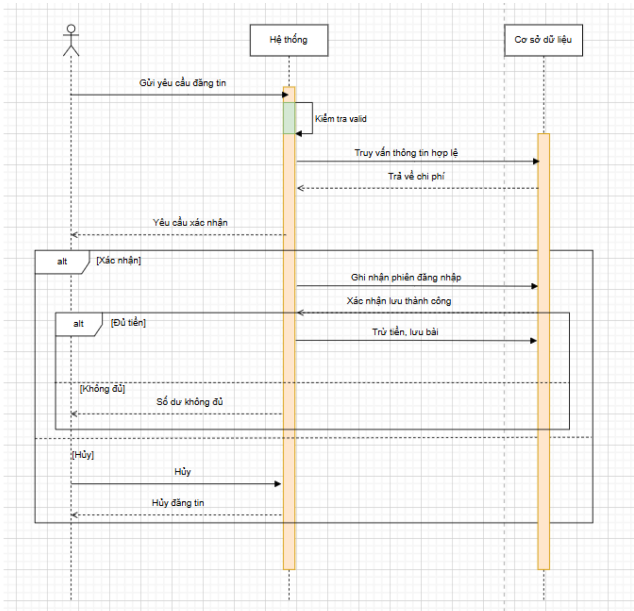
Hình 4.3 Sơ đồ Sequence Đăng tin
