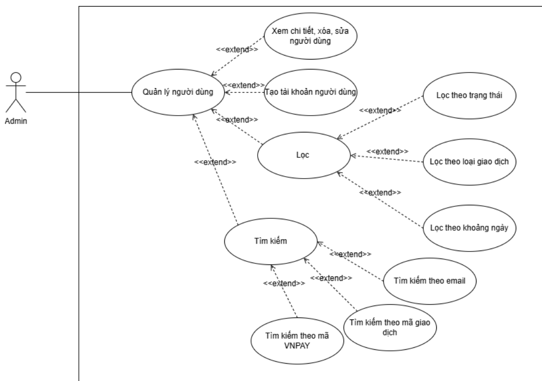
Hình 2.13 Sơ đồ Usecase Quản lý người dùng
