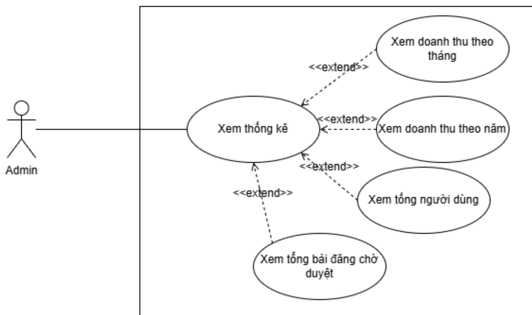
Hình 2.14 Sơ đồ Usecase Xem thống kê
