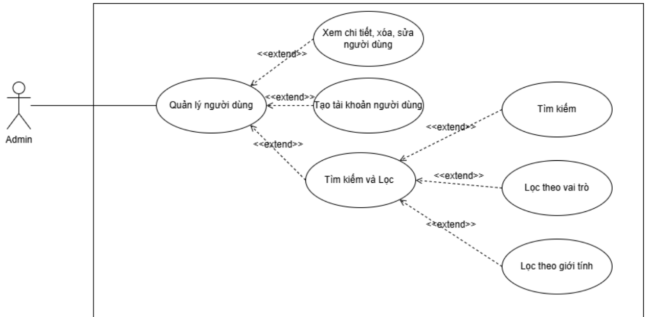
Hình 2.11 Sơ đồ Usecase Quản lý người dùng
