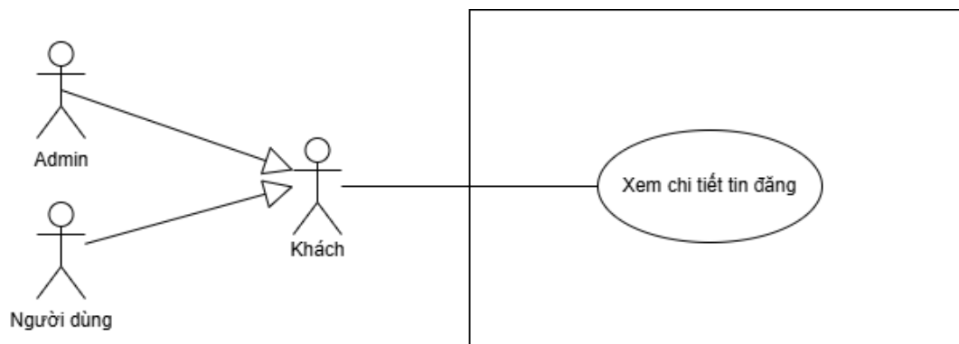
Hình 2.6 Sơ đồ Usecase Xem chi tiết tin đăng
