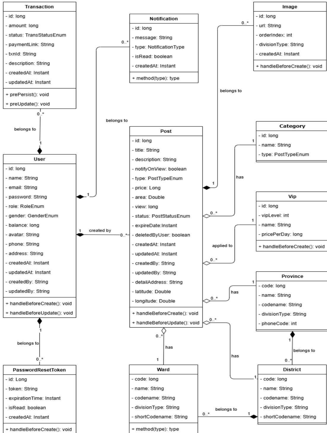
Hình 4.1 Sơ đồ Class Diagram
