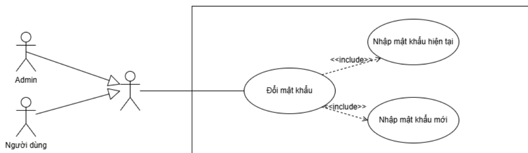
Hình 2.4 Sơ đồ Usecase Đổi mật khẩu
