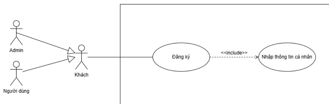
Hình 2.3 Sơ đồ Usecase Đăng ký
