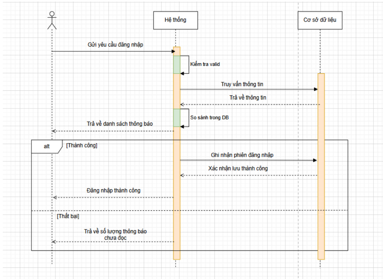
Hình 4.2 Sơ đồ Sequence Đăng nhập
