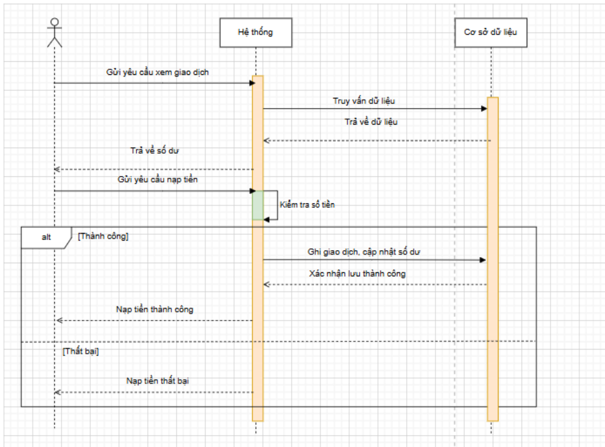
Hình 4.4 Sơ đồ Sequence Thanh toán
