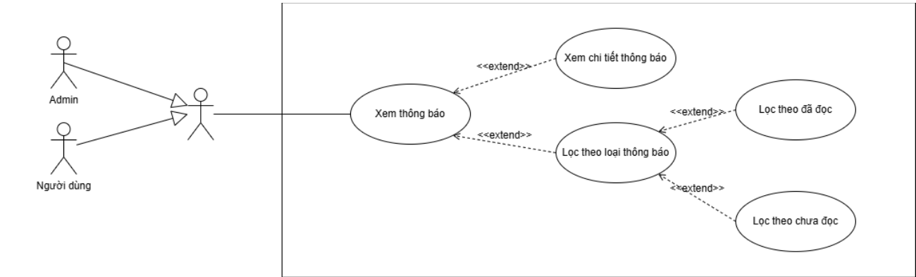
Hình 2.7 Sơ đồ Usecase Thông báo
