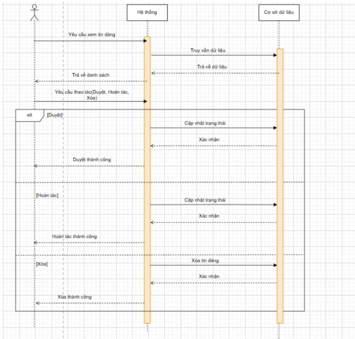
Hình 4.5 Sơ đồ Sequence Quản lý tin đăng
