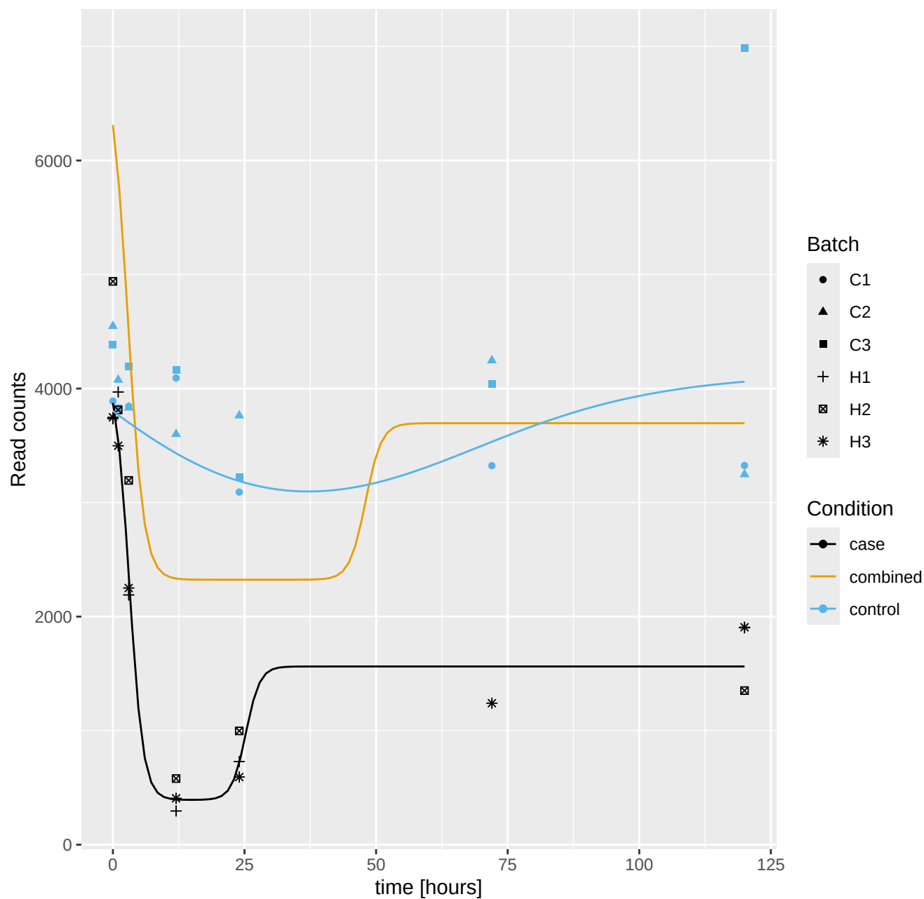
Montipora_capitata_Hlv3__RNAseq.g26807.t1: log10 q = -24.75
