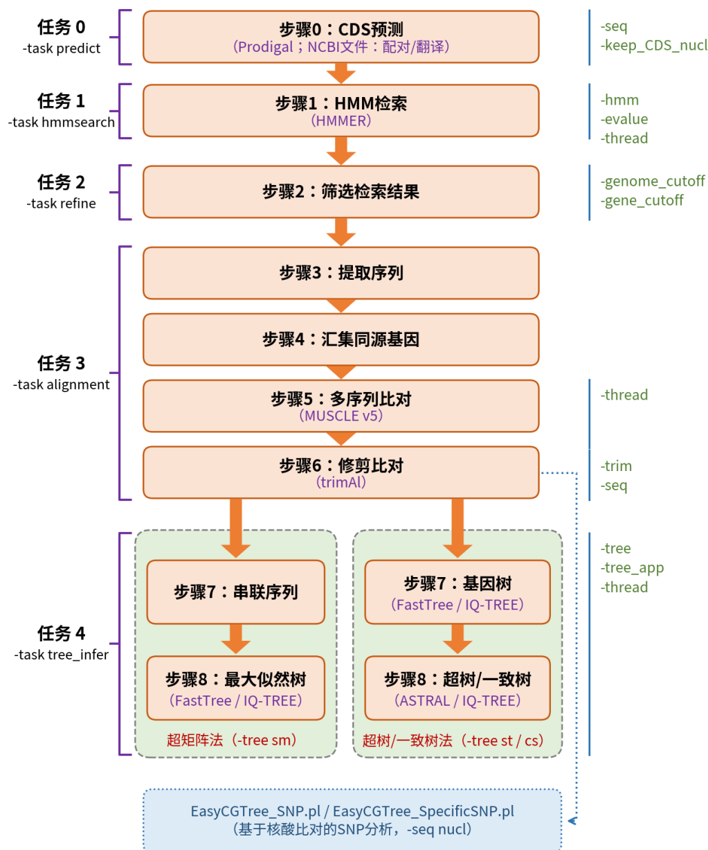
图 2 EasyCGTree 完整运行的流程图
