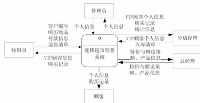
案例- 上下文图
