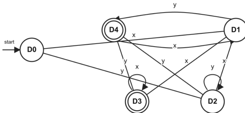
模拟卷07 子集构造 DFA
