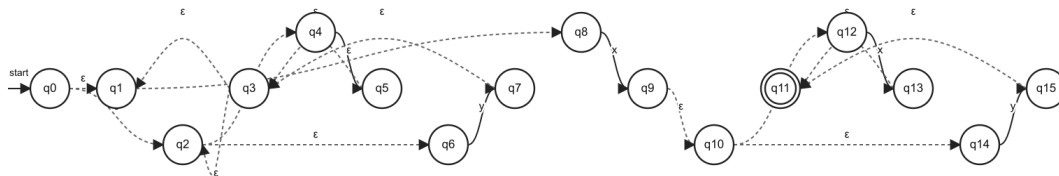
模拟卷07 Thompson NFA
