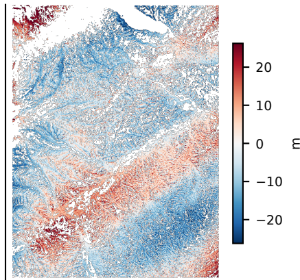
a MintPy OLS DEM error
