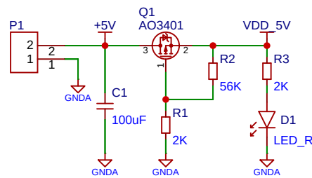
电源输入保护
