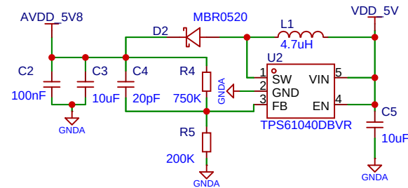
输入电压升压至5.8V
