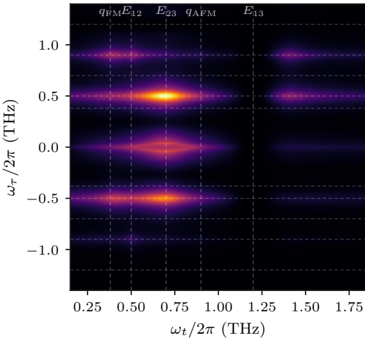
T=0 K
