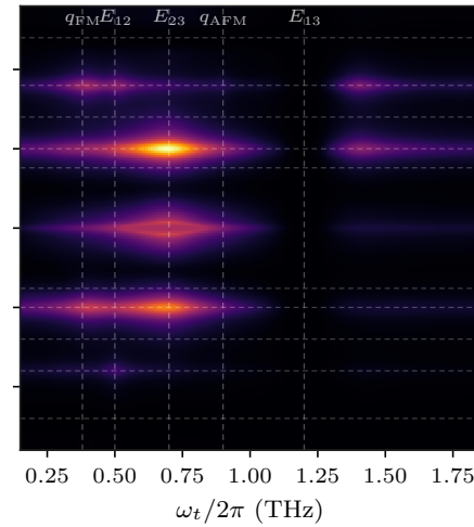
T=20 K
