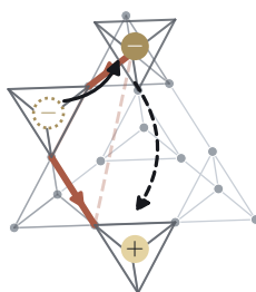
i.b) winding four-loop
