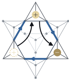
i.a) contractible hexagon
