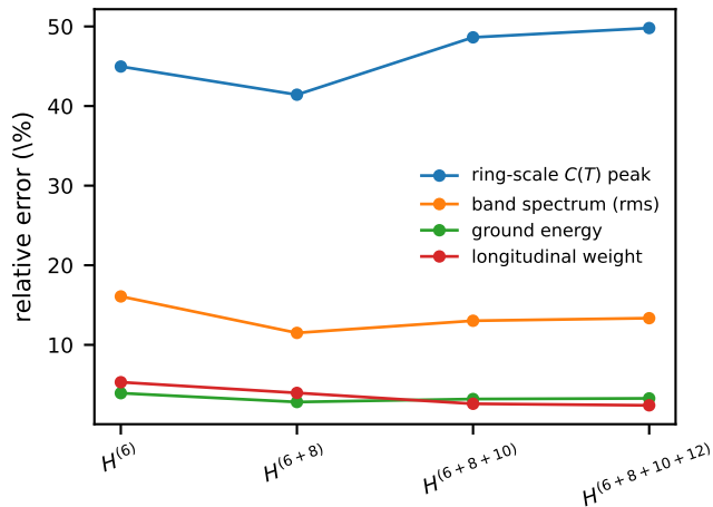
(d) not uniform, at J_{\pm}/J_{zz} = -0.20
