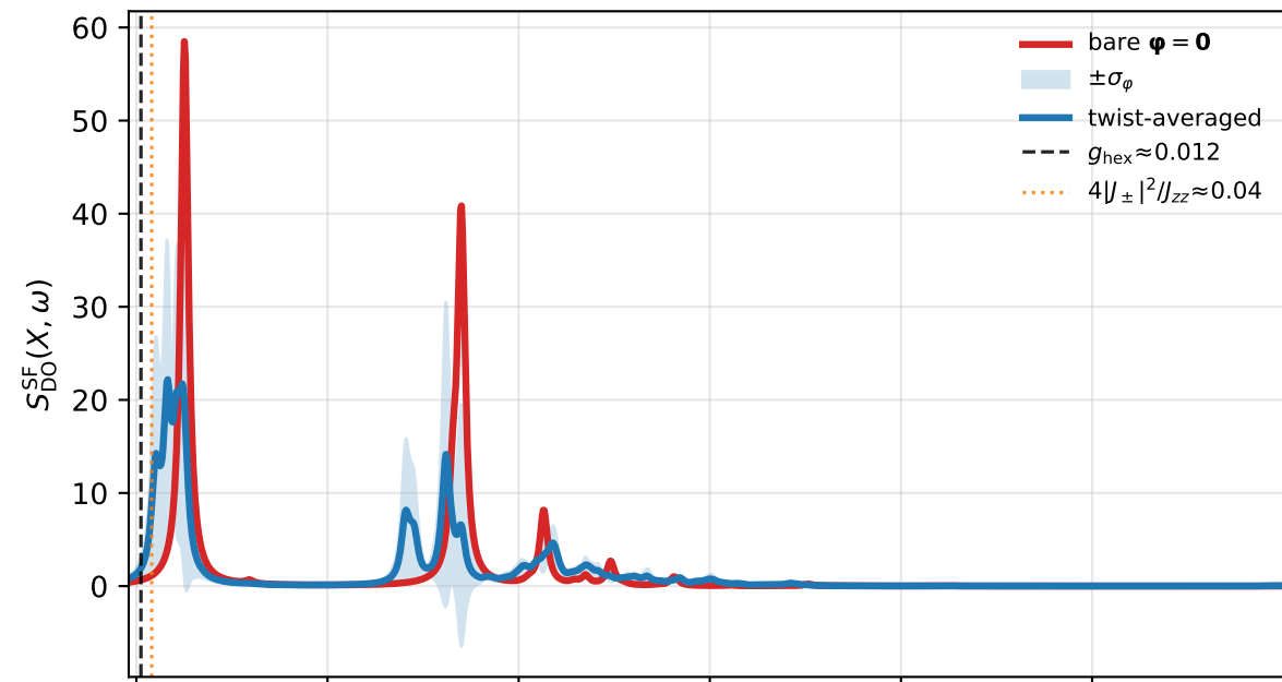
(d) SF, \mathbf{q} = L = (\pi, \pi, \pi)
