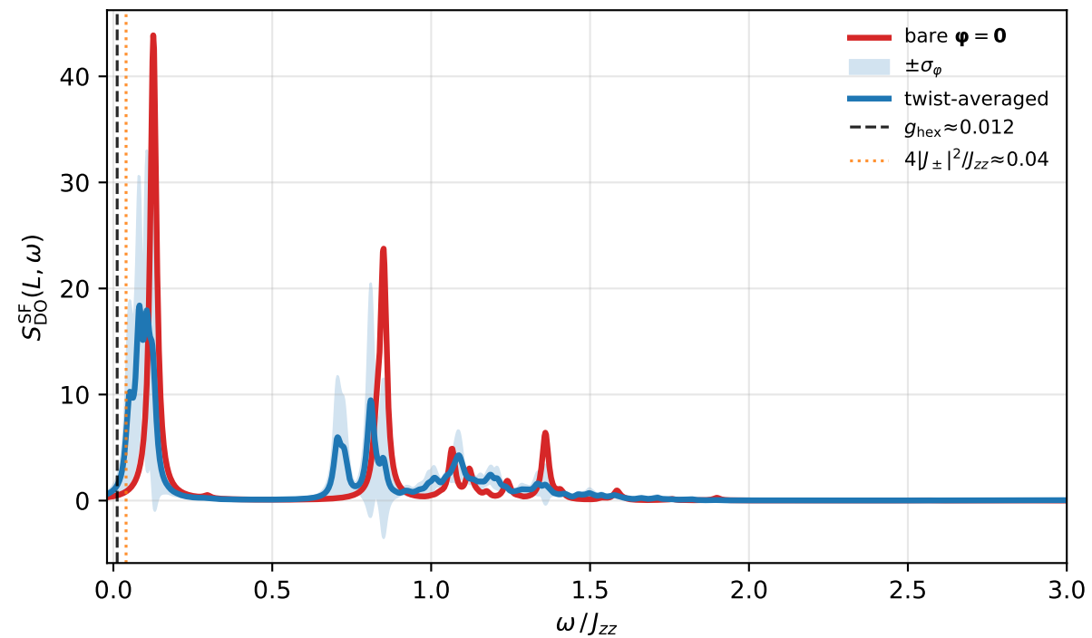
(d) SF, \mathbf{q} = L = (\pi, \pi, \pi)
