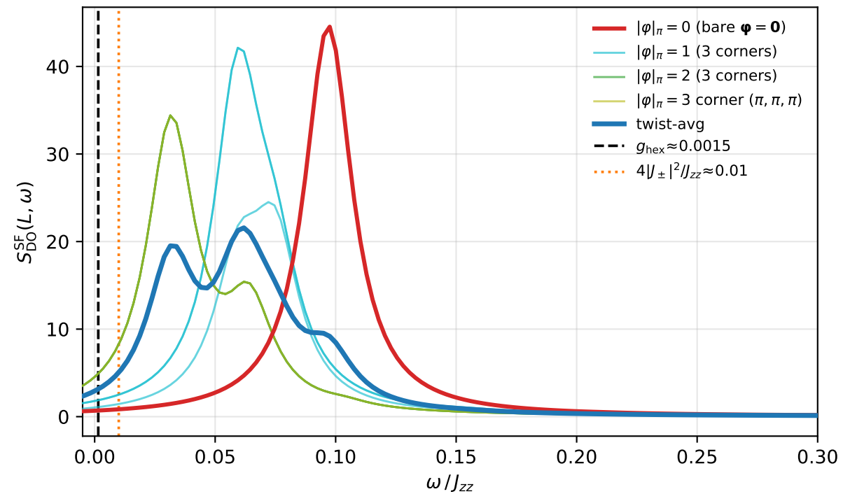
(d) SF, \mathbf{q} = L , low- \omega zoom
