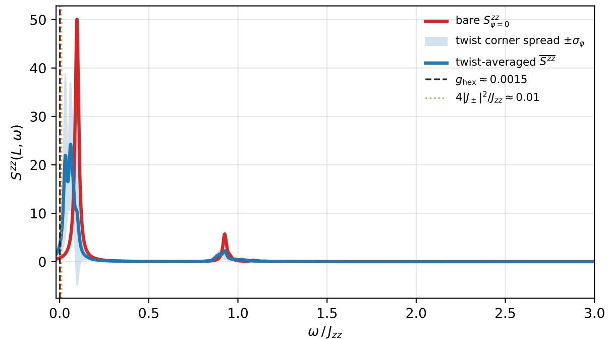
(d) \mathbf{q} = L , bare vs twist-averaged
