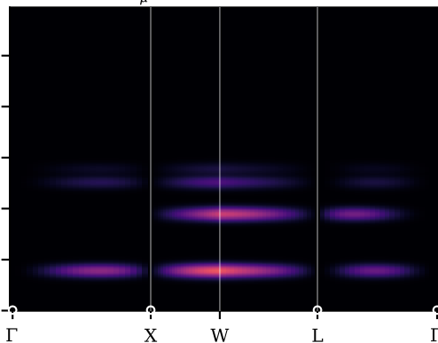
(d) masked, |\sum_{\mu} A^{\mu}|^2 (U(1)-protected)
