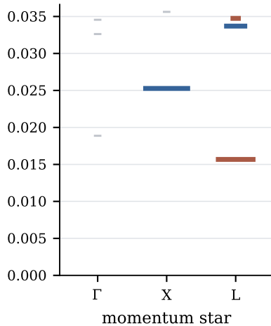
(b) J_{\pm}/J_{zz} = -0.200
