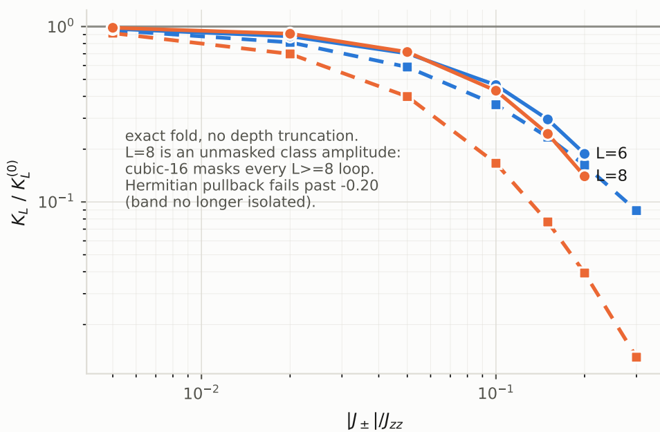
(d) cubic-16: Hermitian (solid) vs Brillouin-Wigner (dashed)
