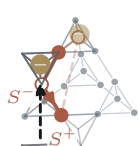
i.f) annihilate
