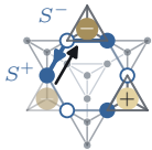
i.b) move
