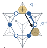
i.c) annihilate
