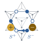
i.a) create
