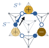
i.b) move
