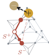
i.f) annihilate
