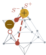
i.d) create
