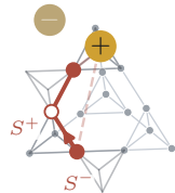
i.e) separate
