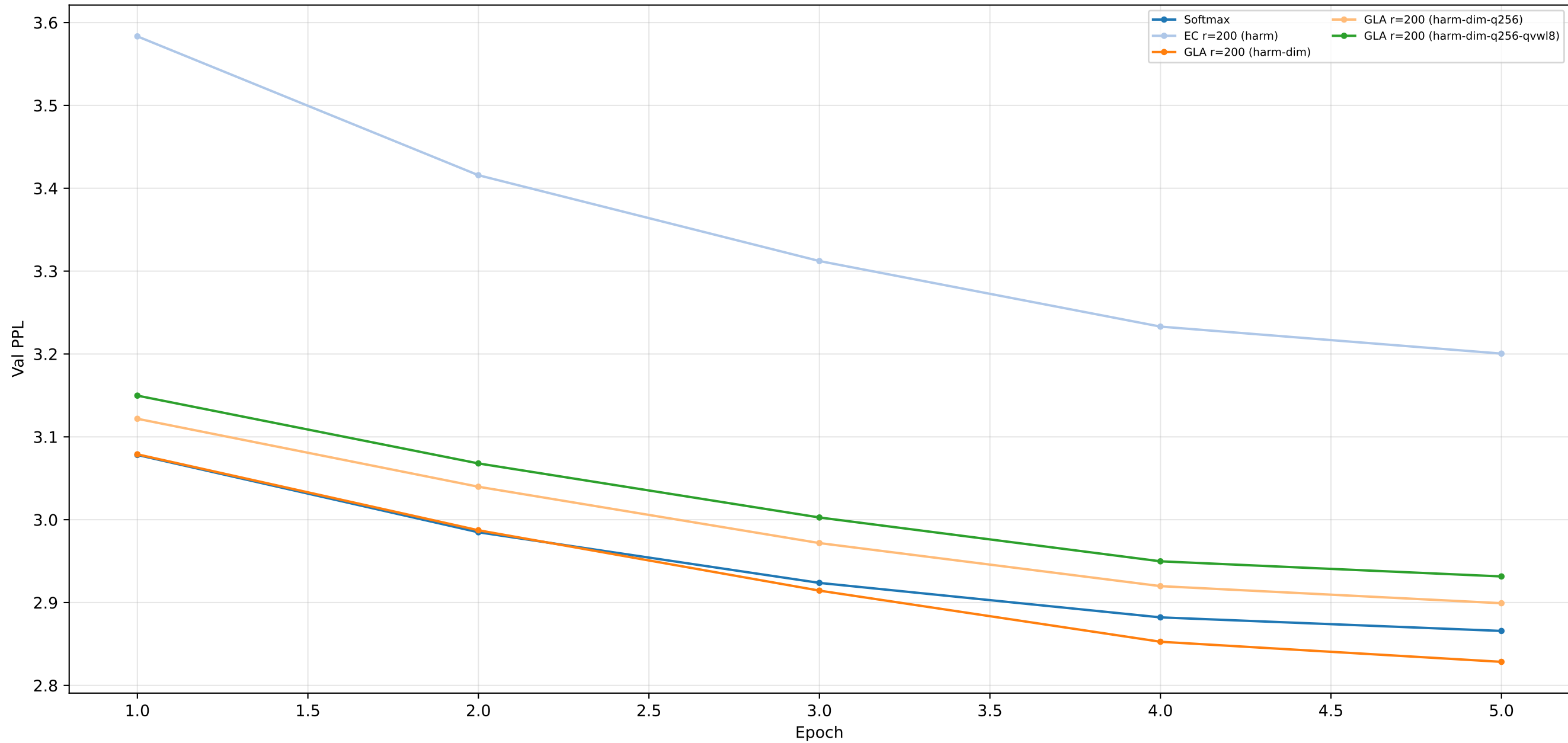
WikiText-103 Validation PPL (seed=42)
