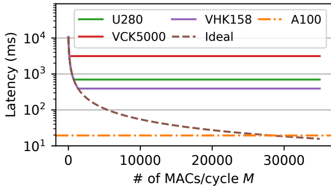
(a) LLaMA2 Prefill Stage
