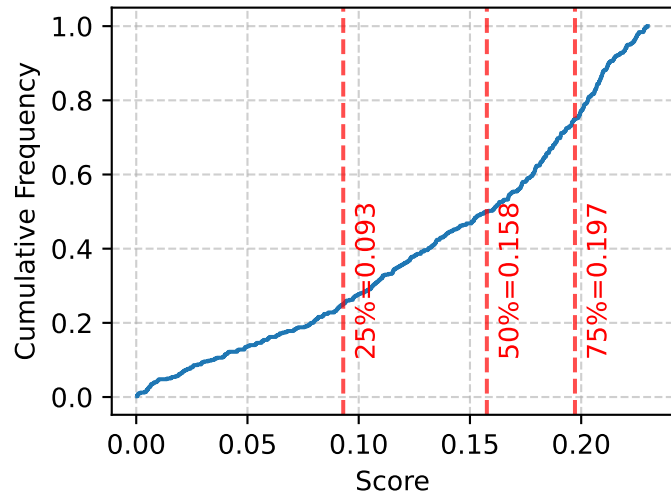
Entropy - MiniLM
