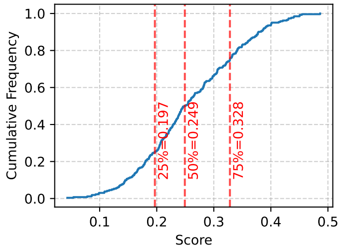
Entropy - MiniLM
