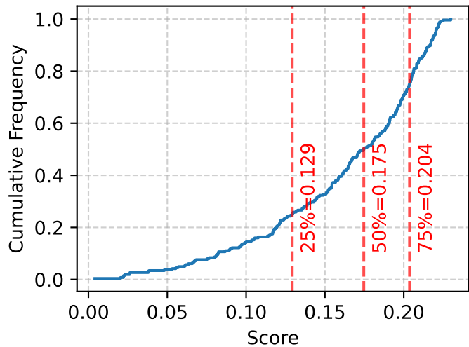
Entropy - MiniLM
