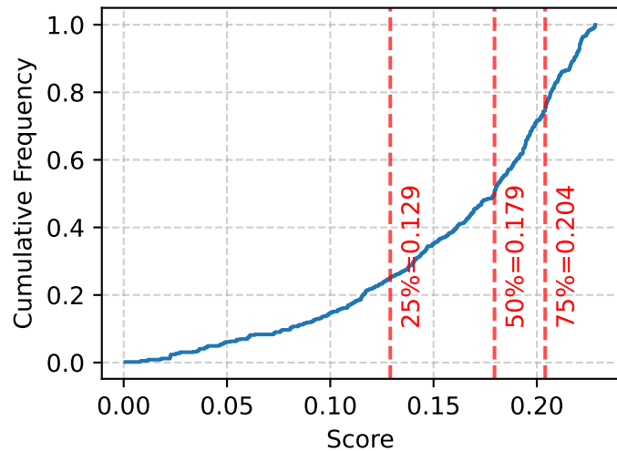
Entropy - 32k
