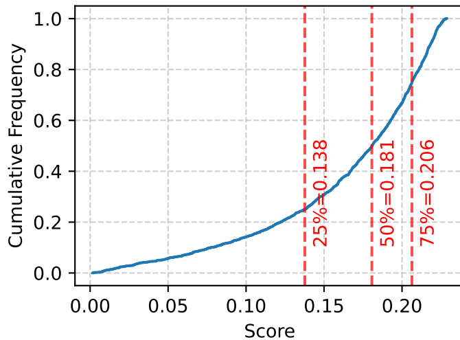
Entropy - 128k
