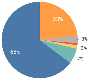
KARL
