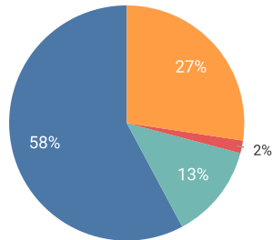
Sonnet 4.5
