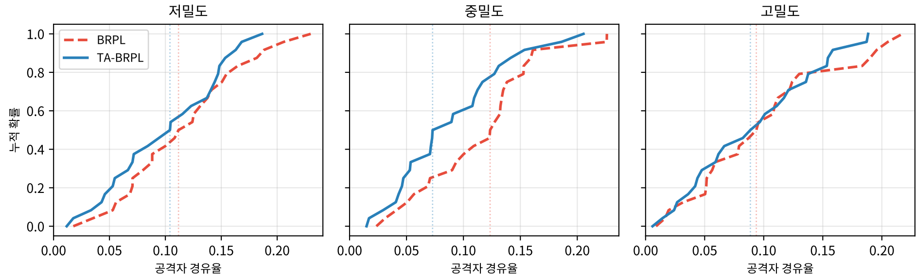
BRPL vs TA-BRPL: 공격자 경유율 누적분포 (각 밀도 25개 토폴로지)
