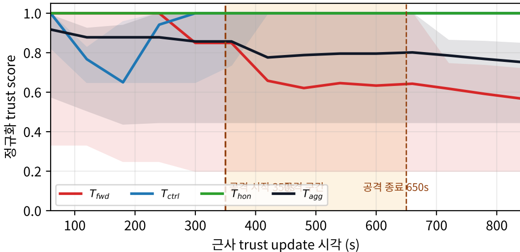
공격자 이웃 trust 신호 시계열 대표 사례: 저밀도 topo_024 ( \Delta att = -0.024 , \Delta churn = +0.000 )
