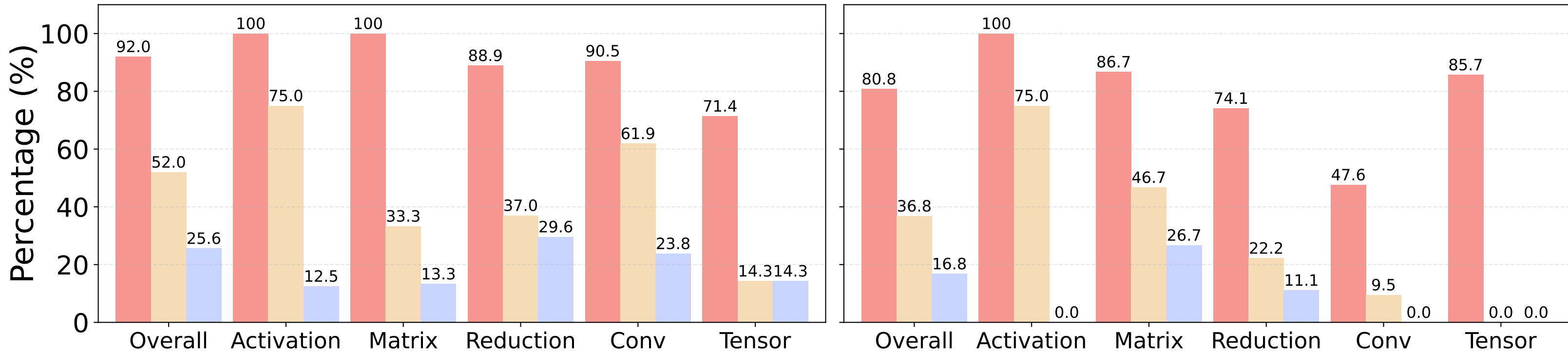
Claude-Sonnet-4.5
