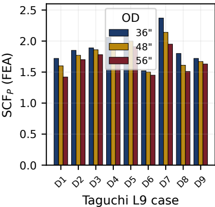
(a) Parametric FEA SCF_P
