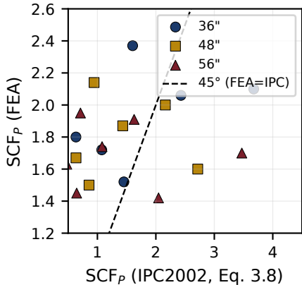
(b) FEA vs IPC2002
