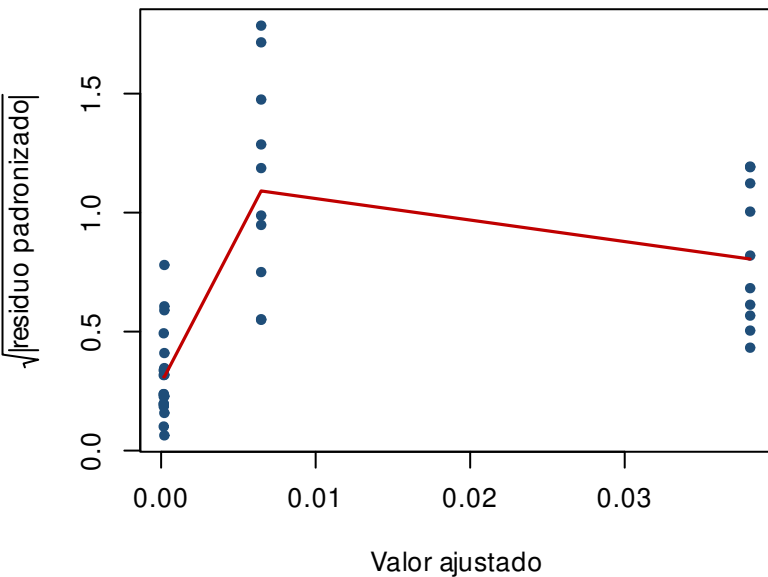
Escala-locacao (homocedasticidade)
