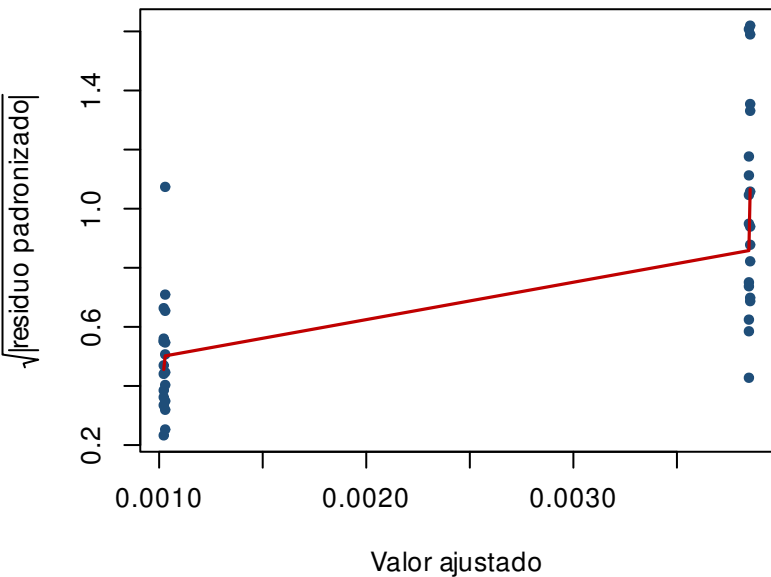
Escala-locacao (homocedasticidade)
