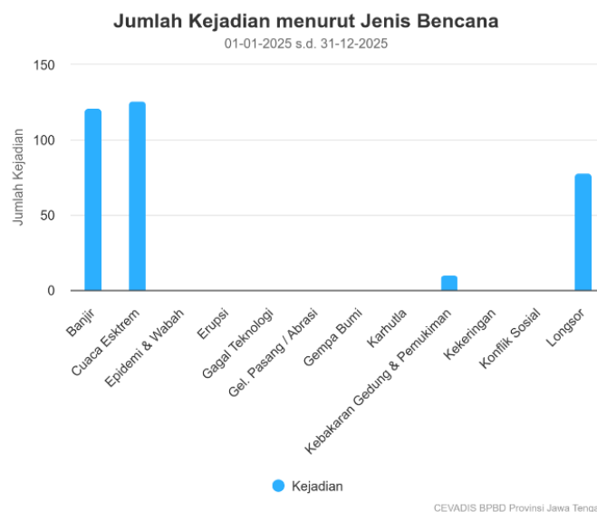
Gambar 2. Jumlah Kejadian menurut Jenis Bencana di Jawa Tengah 2025 Sumber: Badan Penanggulangan Bencana Daerah (BPBD) Provinsi Jawa Tengah, 2025
