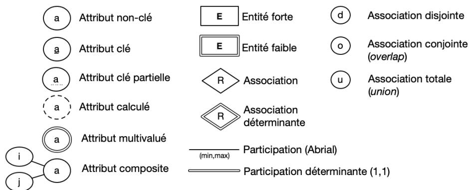
Figure 2. Symboles selon la notation Chen (Elmasri-Navathe)
