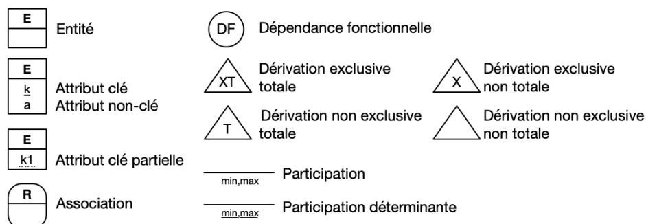
Figure 5. Symboles selon la notation Merise
