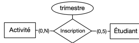
Association déterminante et clé partielle
