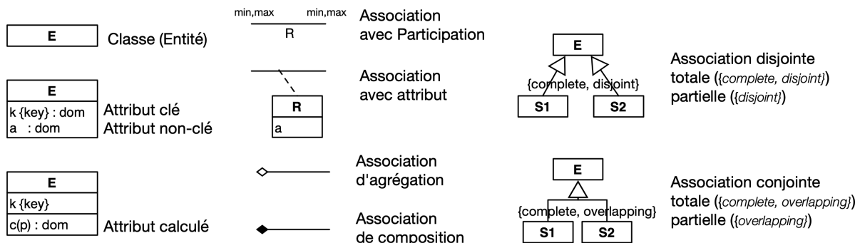
Figure 8. Symboles selon la notation UML
