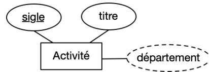
Entité, attribut clé, non clé et calculé
