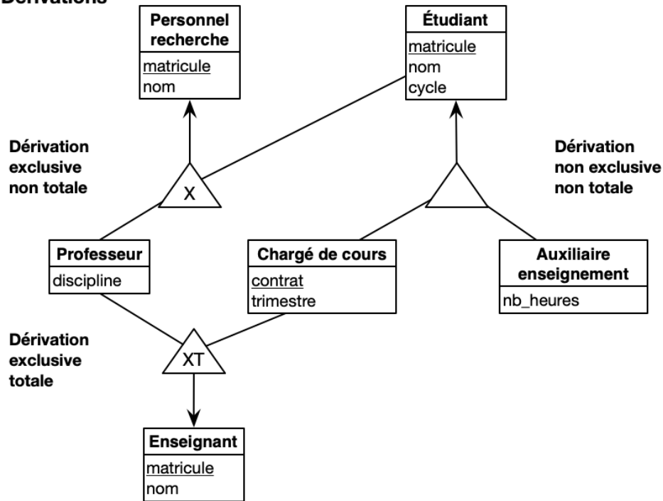
Figure 7. Exemples notation étendue Merise
