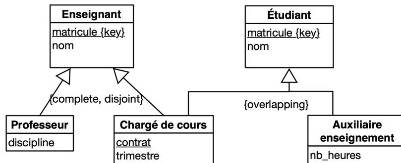
Figure 10. Exemples notation étendue Merise
