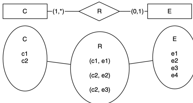
Figure 13. Participation d'une association nécessaire-facultative
