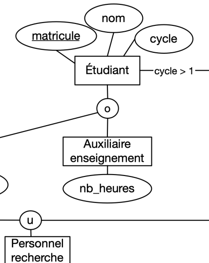
Association par union
