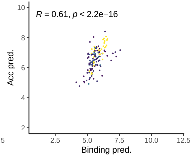
Oct4
