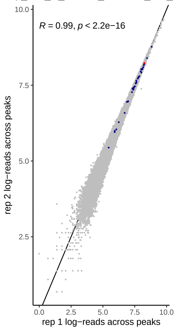
mesc_Btbd11_scenario_WT_coop_mesc
