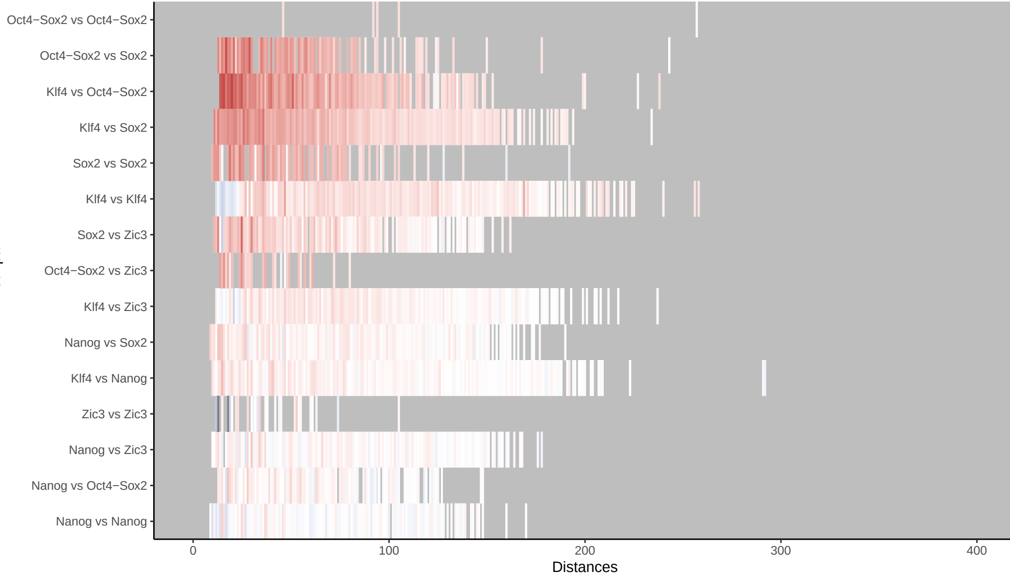
Motif pair
