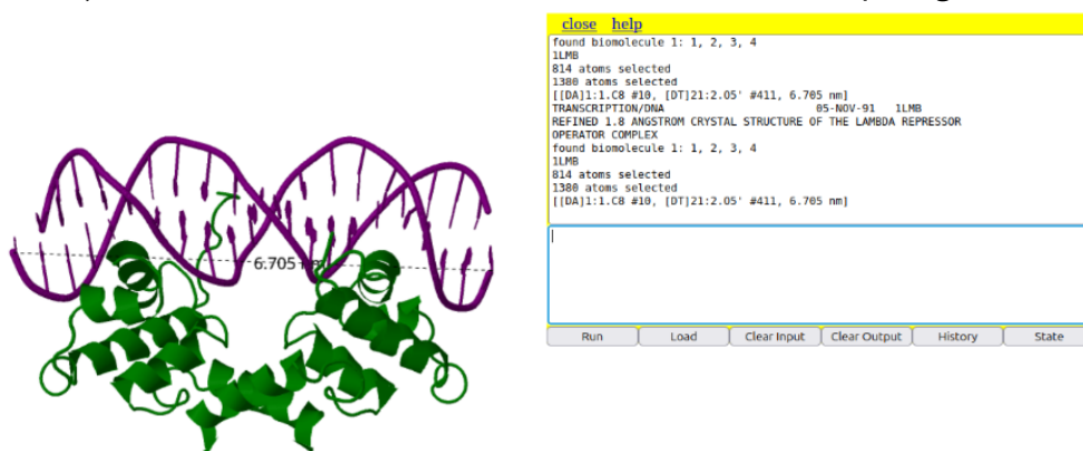
Figura 5: Imagem congelada do JSmol apresentando o complexo opressor-repressor lambda (PDB 1LMB), bem como a medida de seu tamanho, conforme script sugerido no texto.
