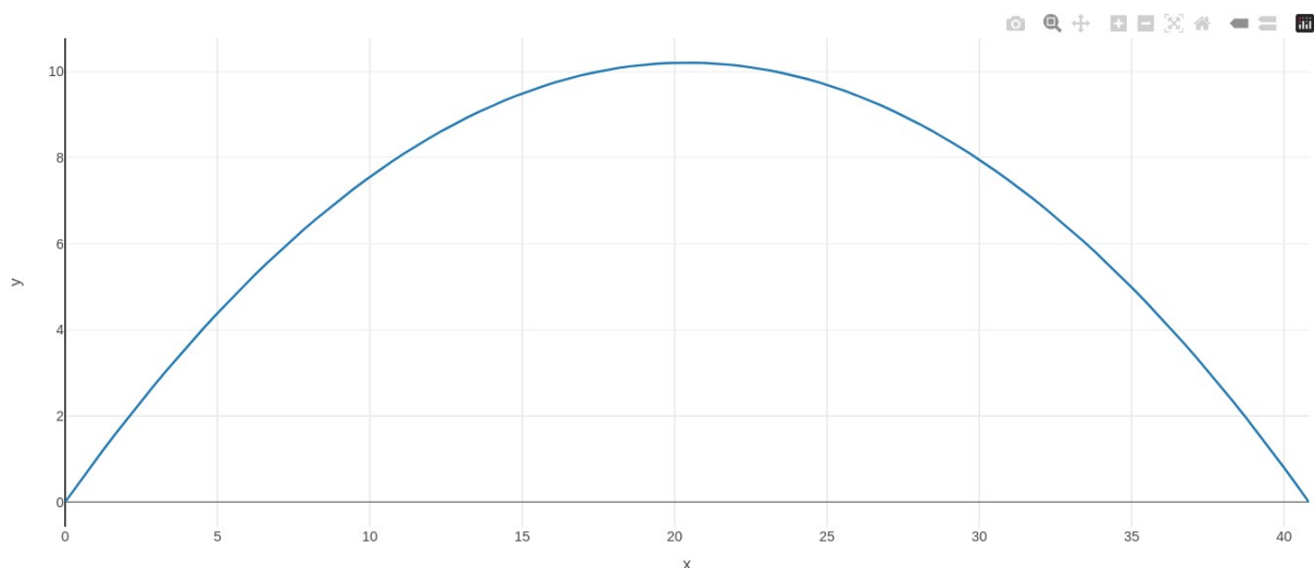
Figura 1: Trajetória parabólica de movimento balístico. Exemplo de um objeto interativo ao ensino reproduível ( OIER ) elaborado com o pacote plotly na plataforma R & RStudio .
