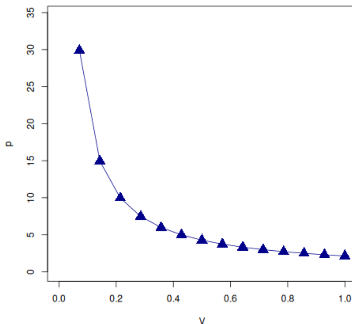
Figura 2: Representação estática de animação de gases ideais conduzida com pacote anim.plots. Para observar a animação, clique neste link .
