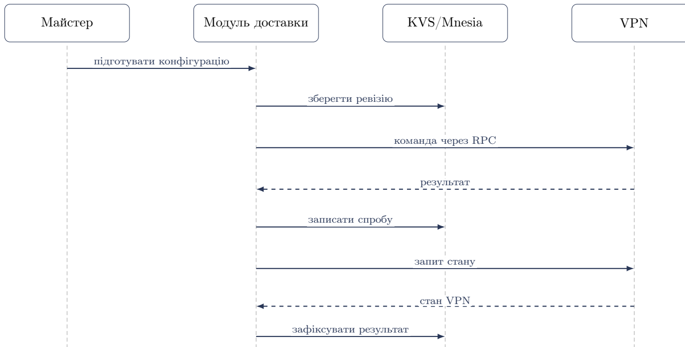
Рис. 4: Послідовність передавання конфігурації та звірення стану
